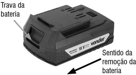
Fig. 6 – Retirando a bateria
