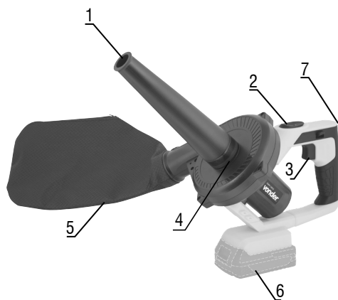
Fig. 1 – Componentes
